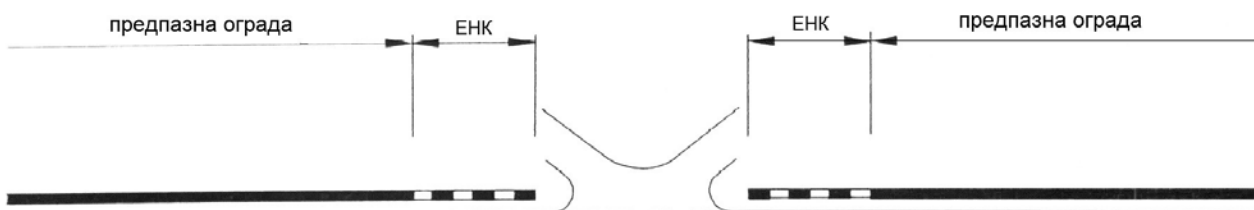
Фигура 11в Прекъсване на скосена 1:12 предпазна ограда със закръгление и ЕНК
