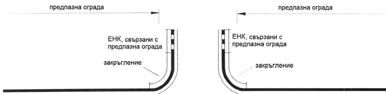
Фигура 11г Прекъсване на предпазна ограда със закръгление и ЕНК
