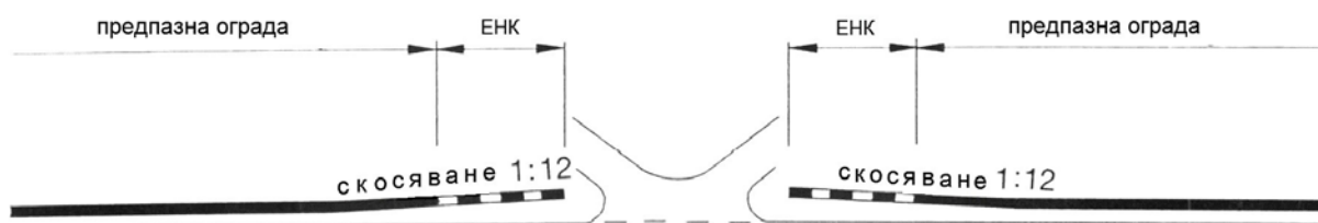
Фигура 11б Прекъсване на предпазна ограда с елементи за начало и край
