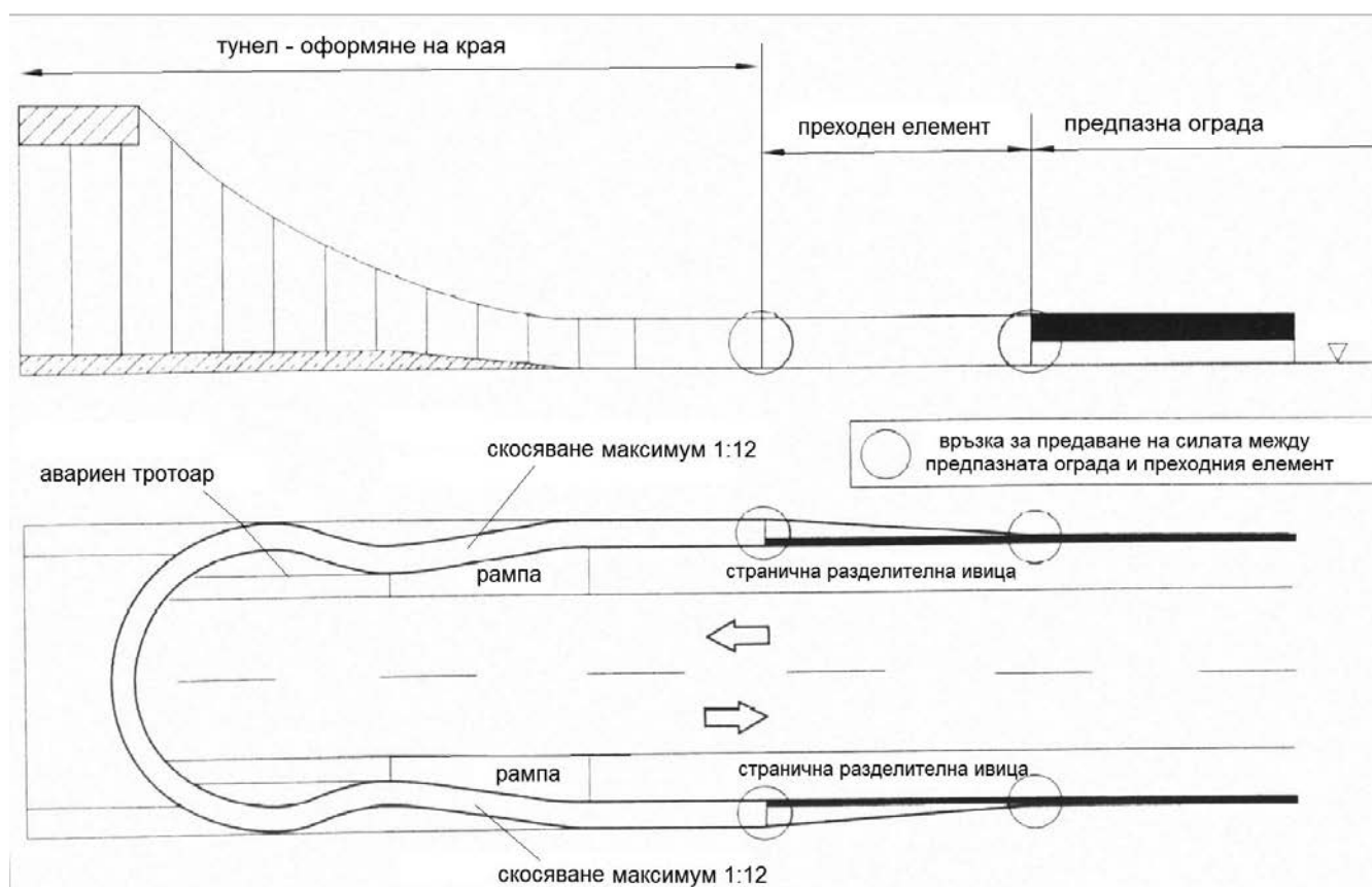
Преходни елементи и предпазна ограда пред тунел
