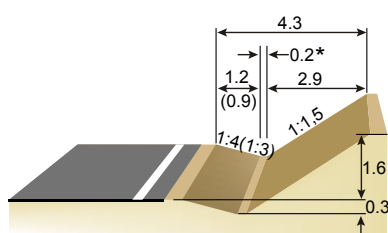
b) side slope gradient 1:1.5
