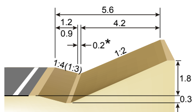
a) side slope 1:2.
